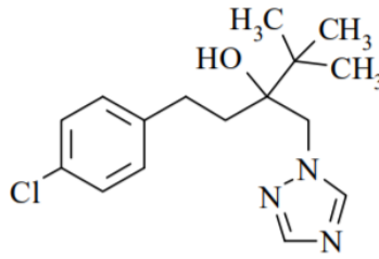
Figura 2.1. Estructura química del tebuconazol.
