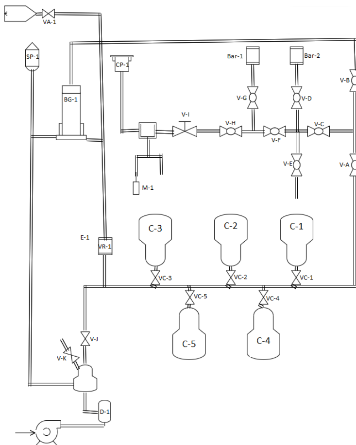
Figura 12 - Esquema de equipo de fisorción
