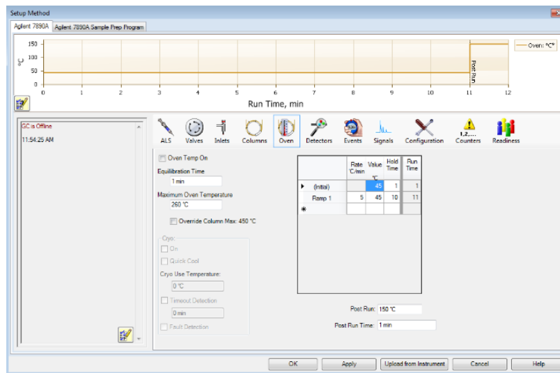
Figura 52 - Ventana de modificación de método (Horno)
