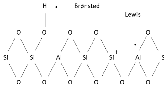
Figura 1 – Sitios ácidos tipo Brønsted y Lewis
