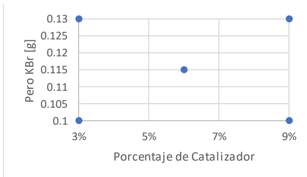
Figura 35 - Plano 2D de datos teóricos
