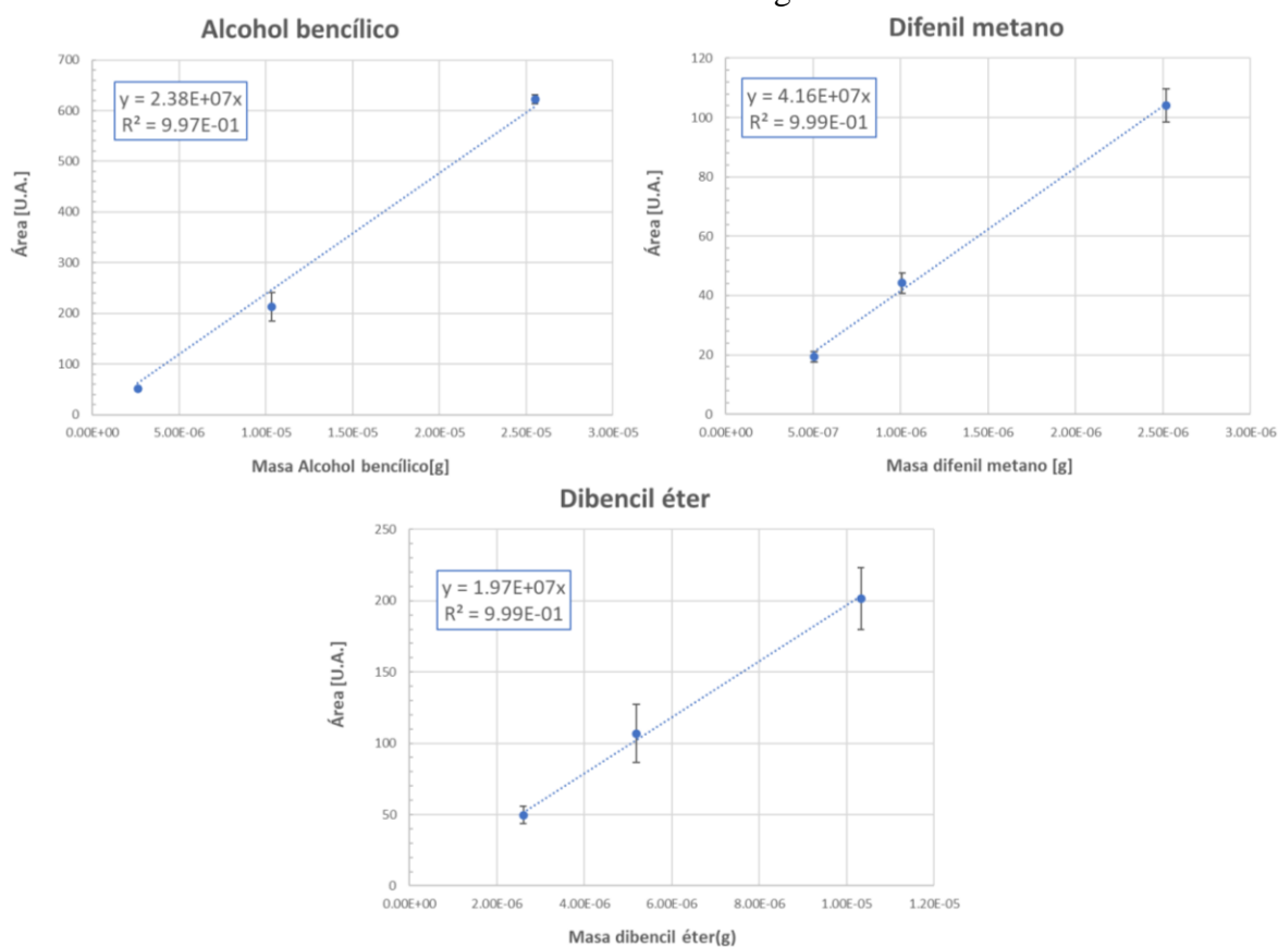
Figura 31 - Calibraciones de reactivos
