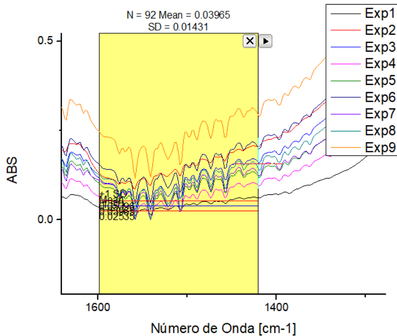
Figura 39 - Análisis de desviación estándar en la zona de 1600 a 1425 cm-1
