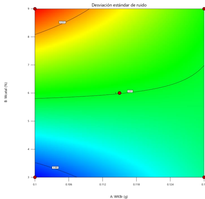
Figura 42 - Zona óptima de disoluciones de KBr y catalizador
