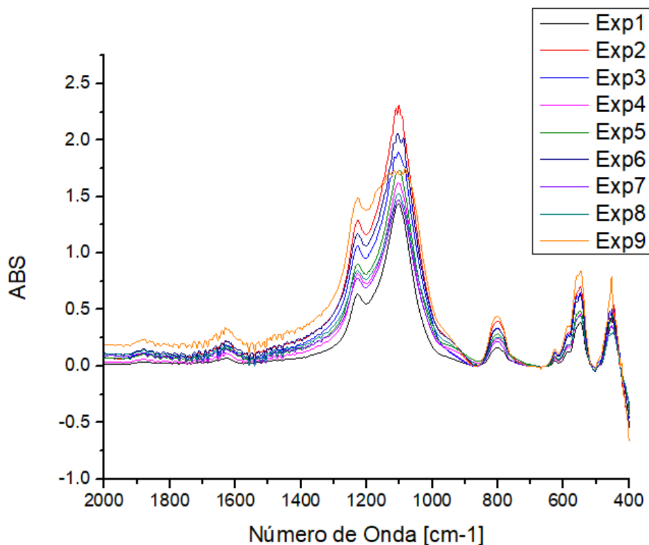
Figura 38 - Comparación de los espectros de infrarrojo de los experimentos 1-9
