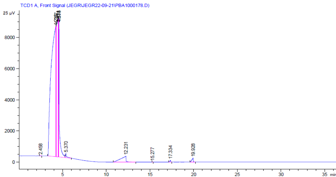
Figura 30 - Cromatograma de HZW30 tras 7 horas de reacción
