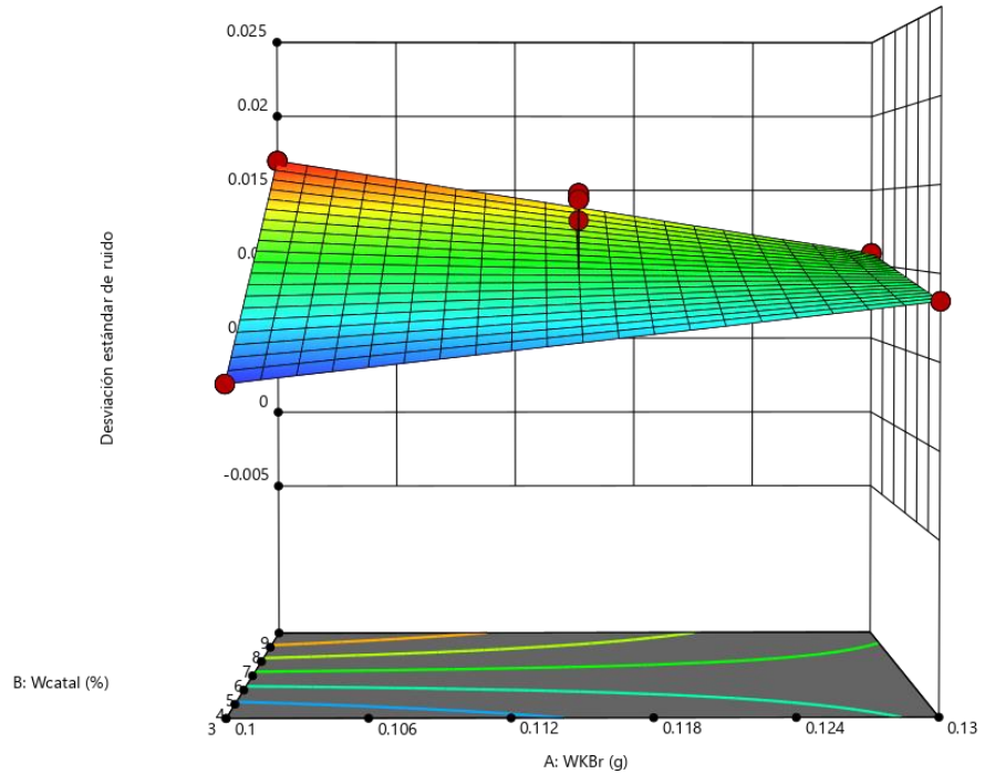
Figura 40 - Gráfica 3D de ruido en función de las disoluciones de KBr y catalizador.
