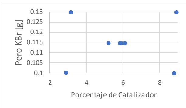
Figura 36 - Plano 2D de datos experimentales
