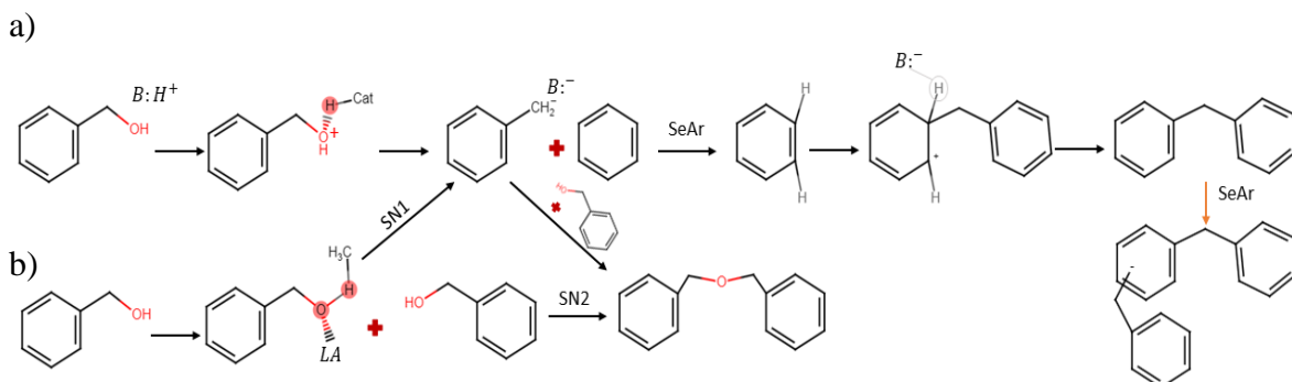
Figura 33 - Mecanismos de reacción propuestos para la generación de a) DFM y b) DBE
