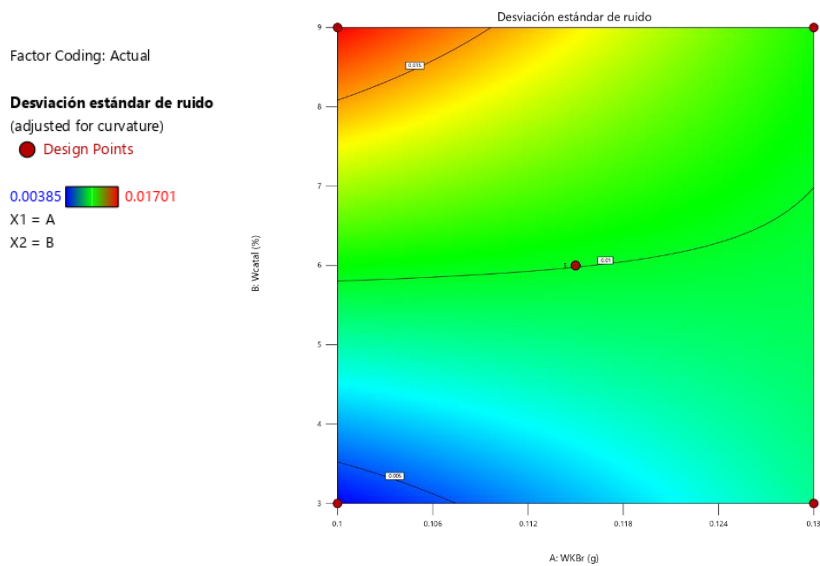
Figura 41 - Gráfica 2D de ruido en función de las disoluciones de KBr y catalizador
